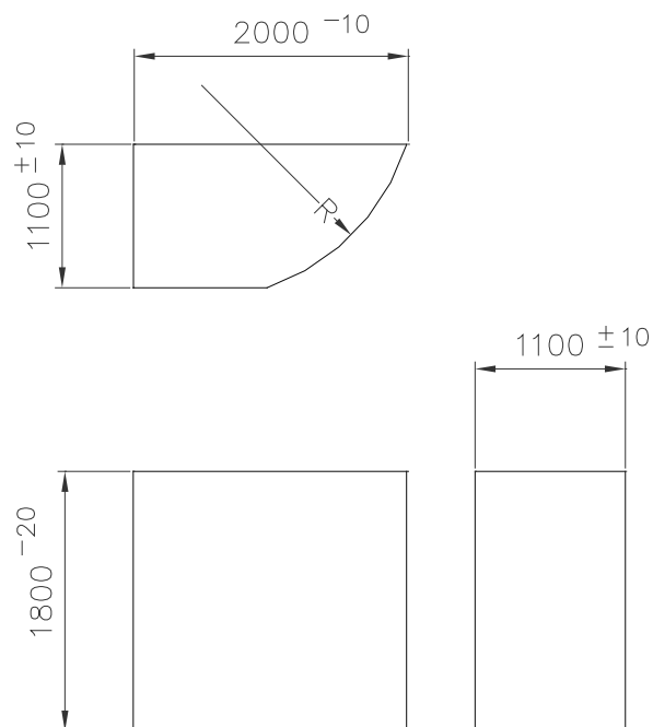
Rys.4. Komora powłoki - wymiary gabarytowe
