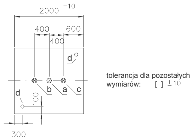
Rys. 6. Komora powłoki - widok z góry. Układ zaworów i króćców.
