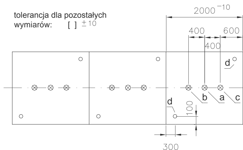
Rys. 3. Powłoka - widok z góry. Układ zaworów i króćców.
