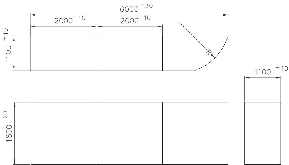
Rys. 1. Powłoka z podziałem na komory - wymiary gabarytowe
